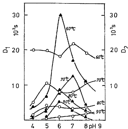
Abb. 2. Einfluß des pH-Wertes auf die Inaktivierungsgeschwindigkeit von Meerrettichperoxidase bei verschiedenen Temperaturen. \odot D_1 : aus den steilen Kurventeilen, \blacktriangle D_2 : aus den flachen Kurventeilen.
